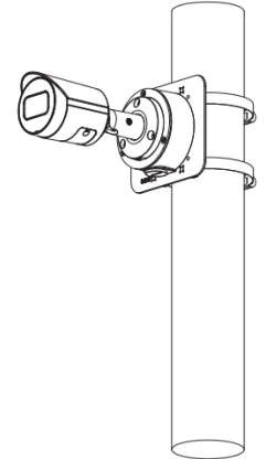
PFA134+PFA152-E 立柱安裝
