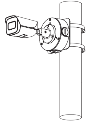
PFA130-E+PFA152-E 立柱安裝
