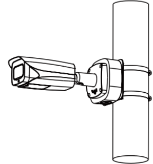
PFB121 + PFA152 立柱安裝
